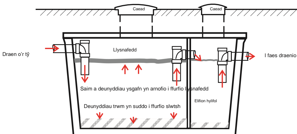
Ffigur 1: enghraifft o danc septig (h) Eryri-Bywiol
