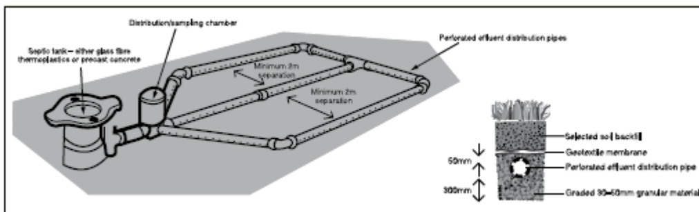
Ffigur 2: enghraifft o maes draenio nodweddiadol (Adran H2 y Rheoliadau Adeiladu)
